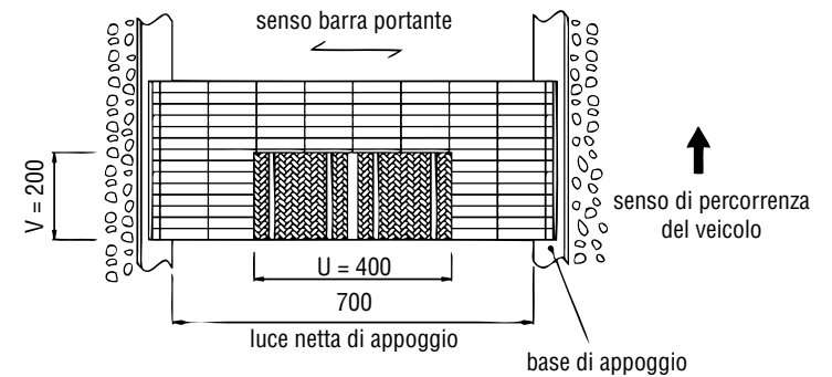
Schema di calcolo
