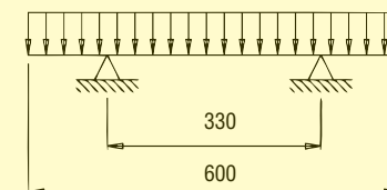
Schema di calcolo
